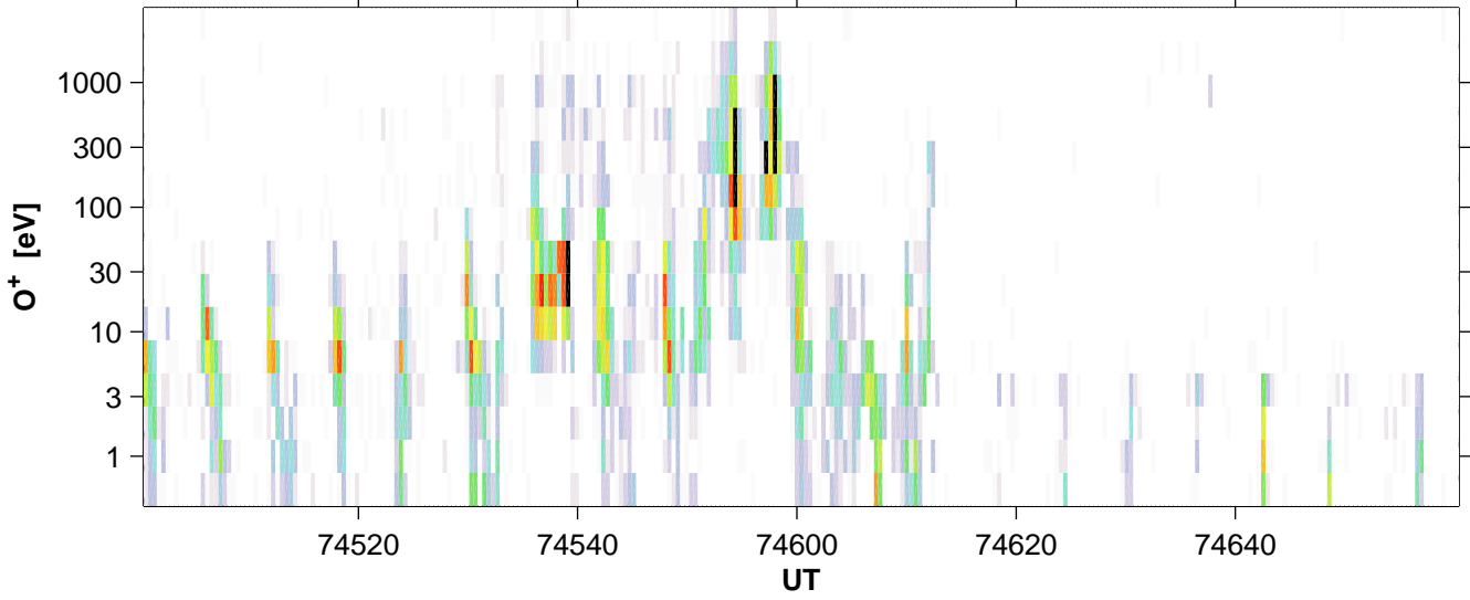
Freja Orbit: 1718
