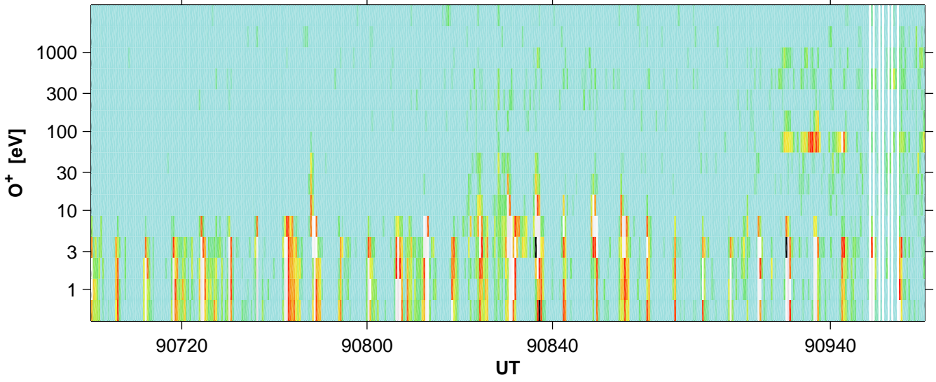
Freja Orbit: 5948
